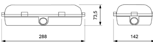
Montaje estanco
